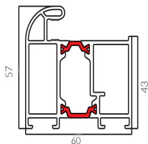
Ościeżnica „TERMO do EXPERT 64”
