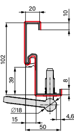
OŚCIEŻNICA STALOWA NAROŻNA
