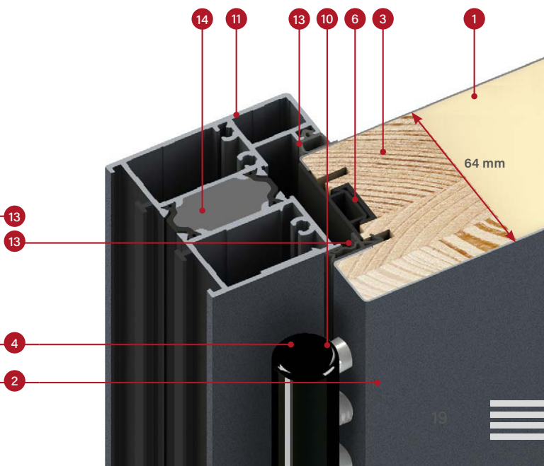
przekrój ościeznicy stalowej dla skrzydła THERMO 64
